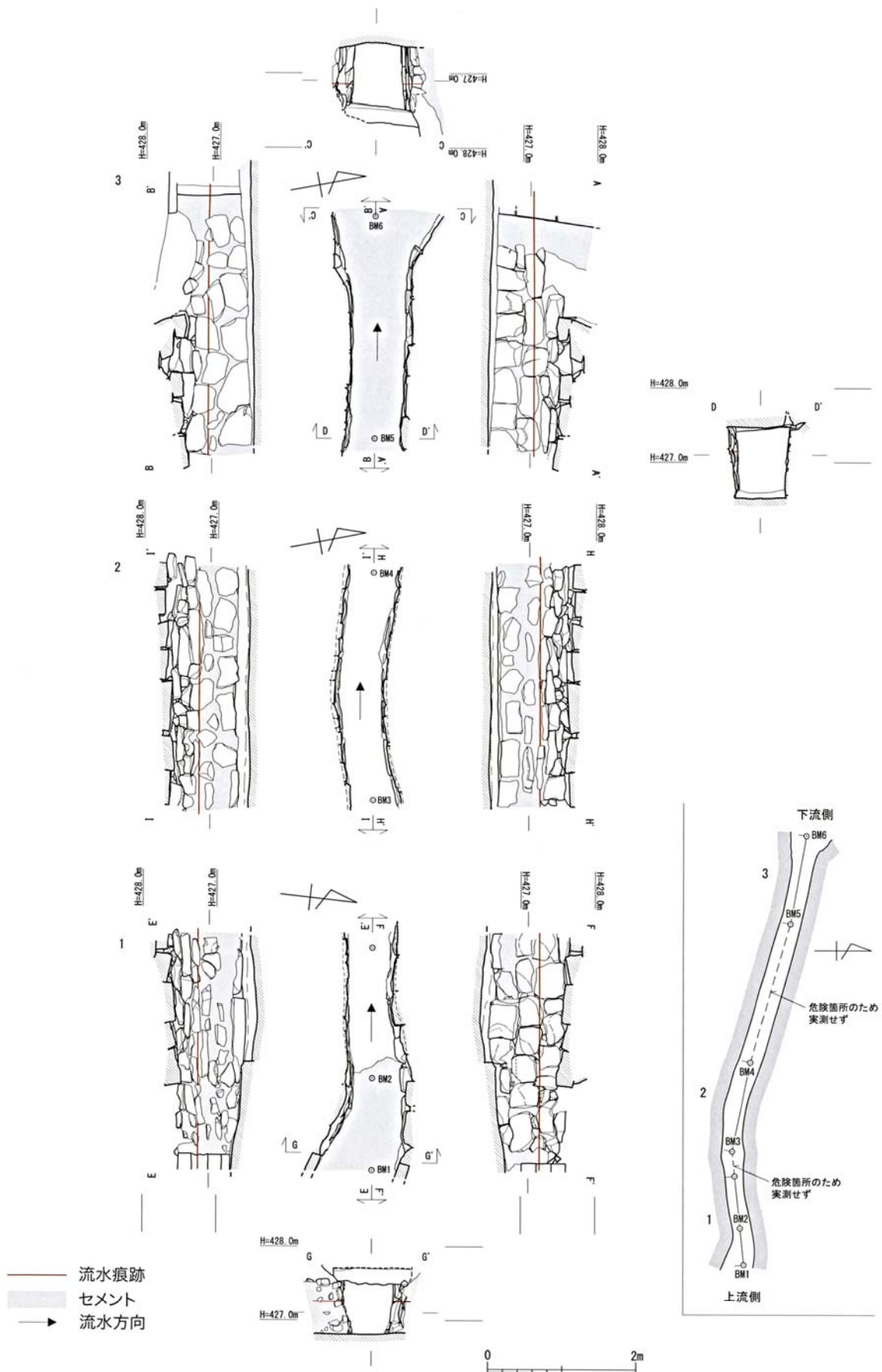
図(PL)36 通潤用水下井手16号水路 石組隧道(S=1/80)
