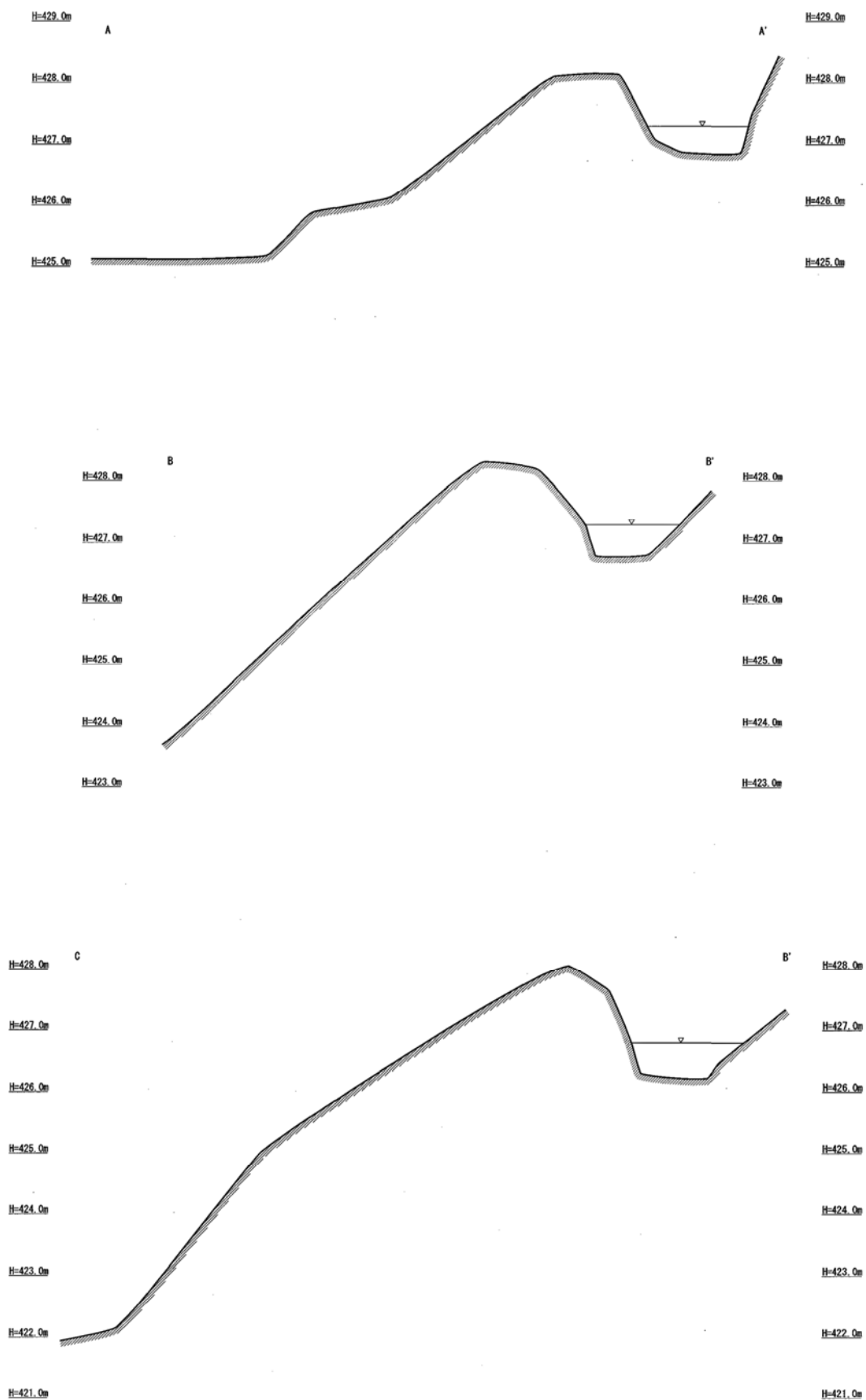
図(PL)39 通潤用水下井手18号水路 横断面図(S=1/100)
