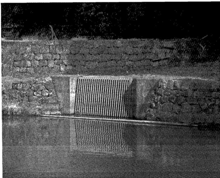
写真(PL)5 下井手取水口
