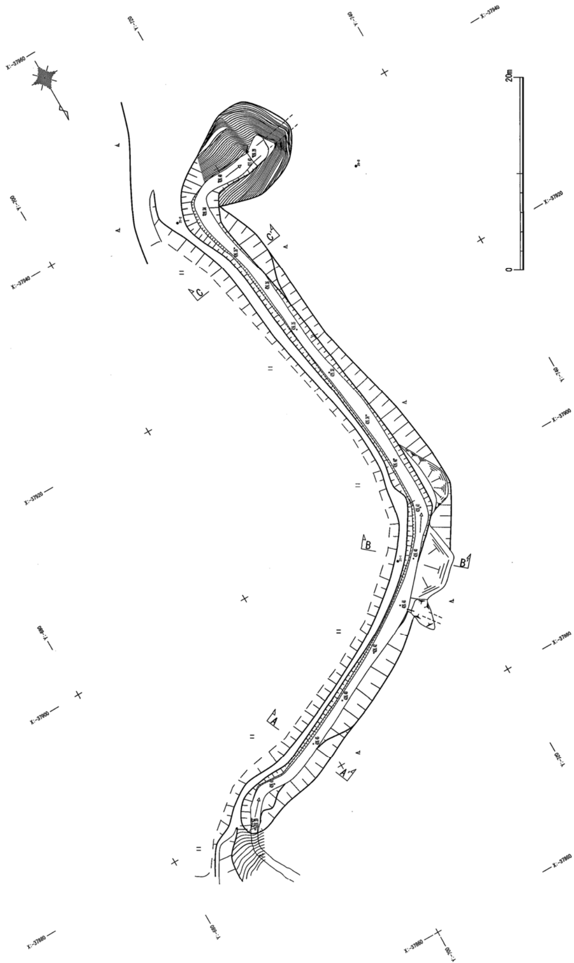
图 (PL) 42 通潤用水下井手21号水路 平面图 (S=1/400)
