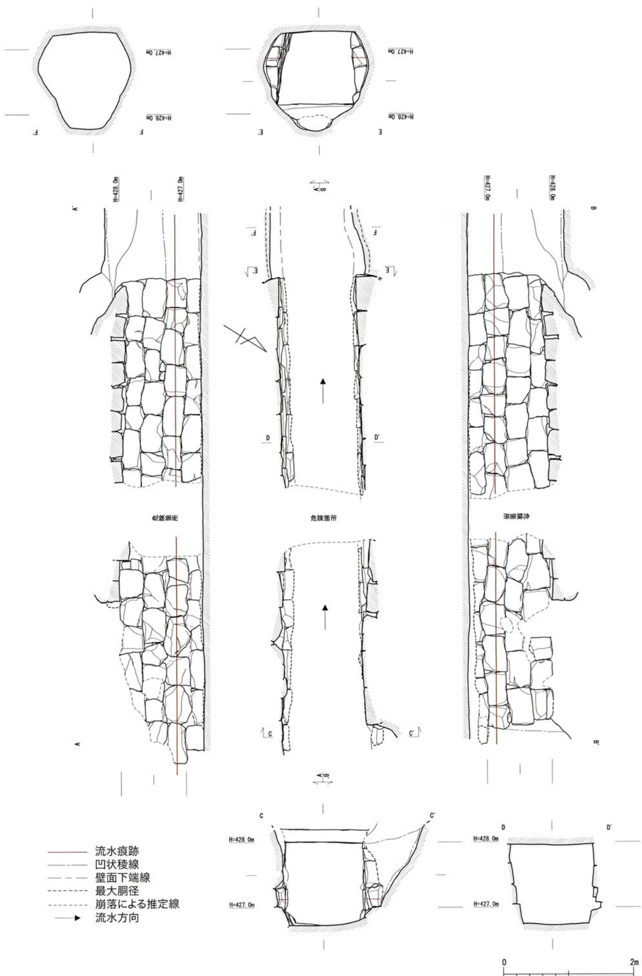
図(PL)41 通潤用水下井手18号水路 下流坑口 (S=1/60)
