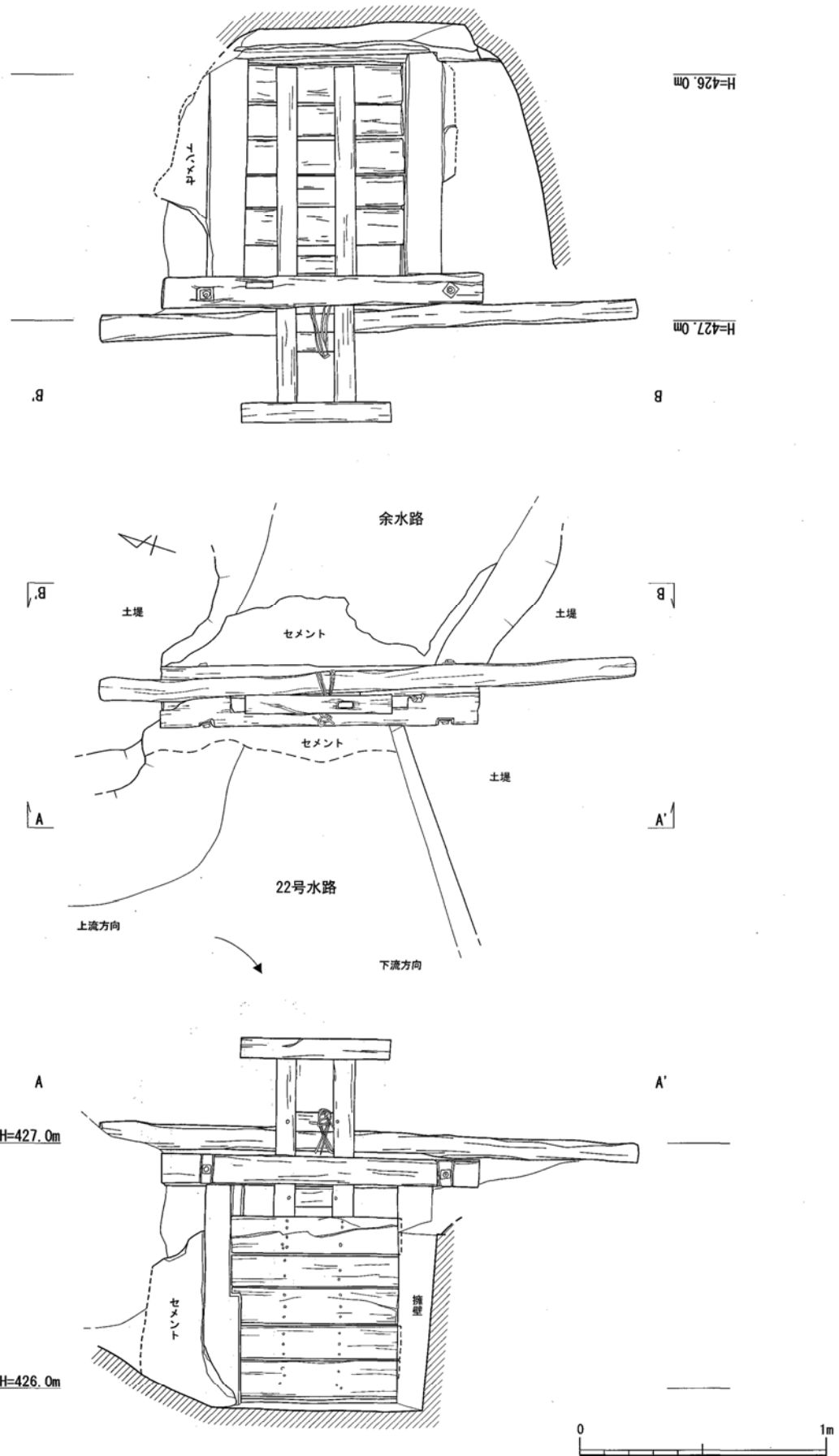
図(PL)49 通潤用水下井手22号水路 余水吐(S=1/25)
