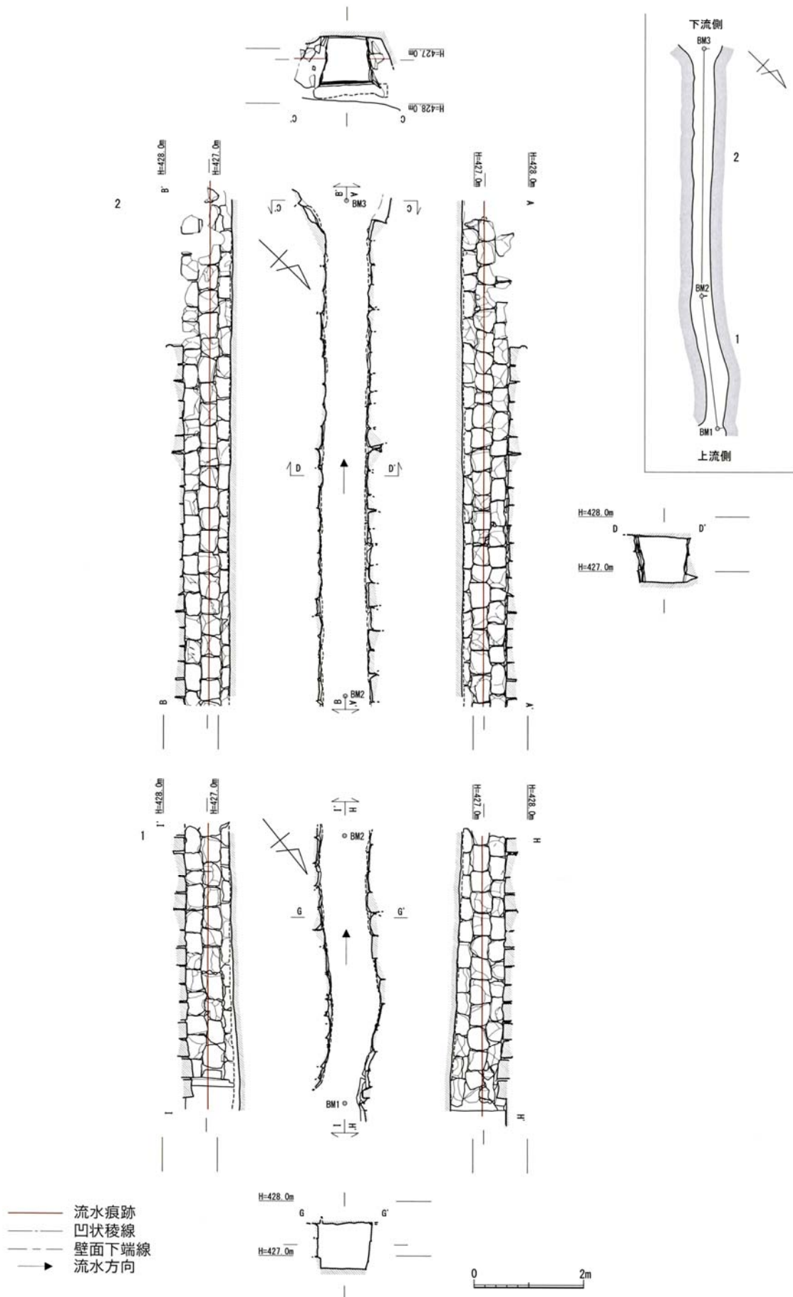
図(PL) 40 通潤用水下井手18号水路 石組隧道(S=1/100)
