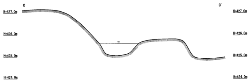
図(PL)52 通潤用水下井手24・25号水路 横断面図(S=1/100)
