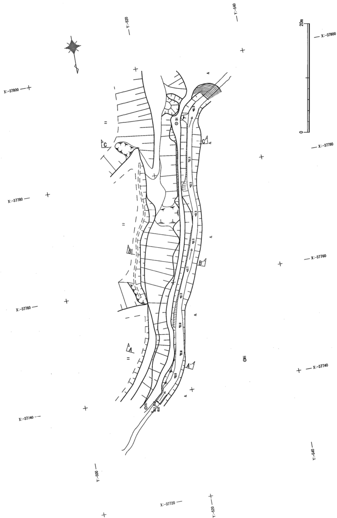
图(PL)37 通潤用水下井手18号水路 平面图(S=1/400)
