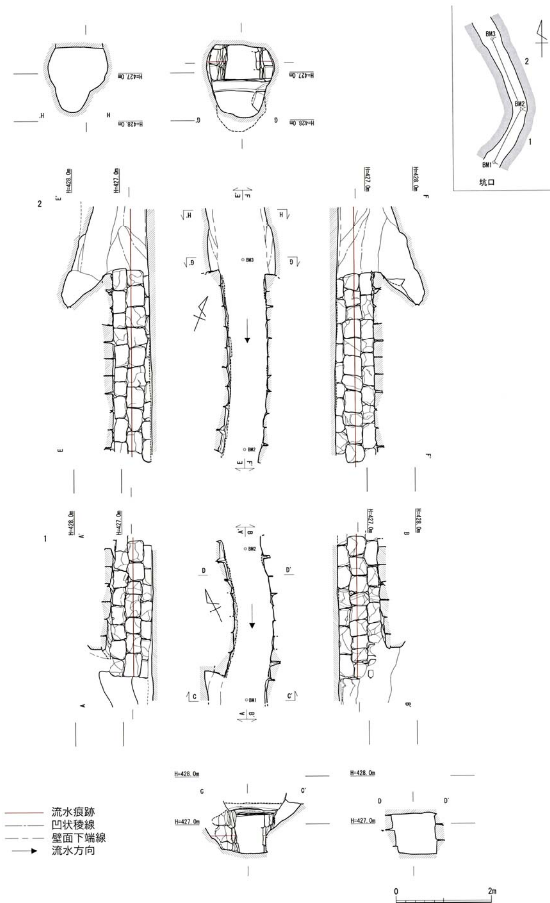
図(PL) 45 通潤用水下井手21号水路 上流坑口(S=1/80)
