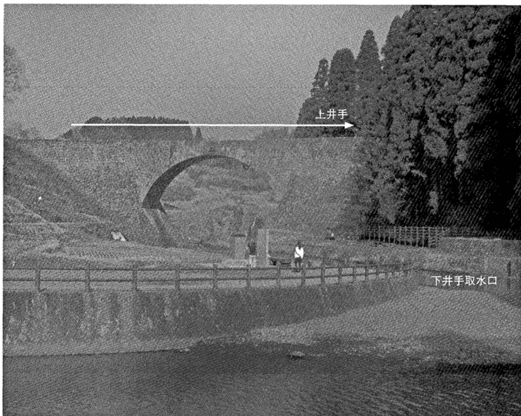
写真(PL)2 通潤橋 橋の通水管内部を上井手が流れる. 右下は下井手取水口
