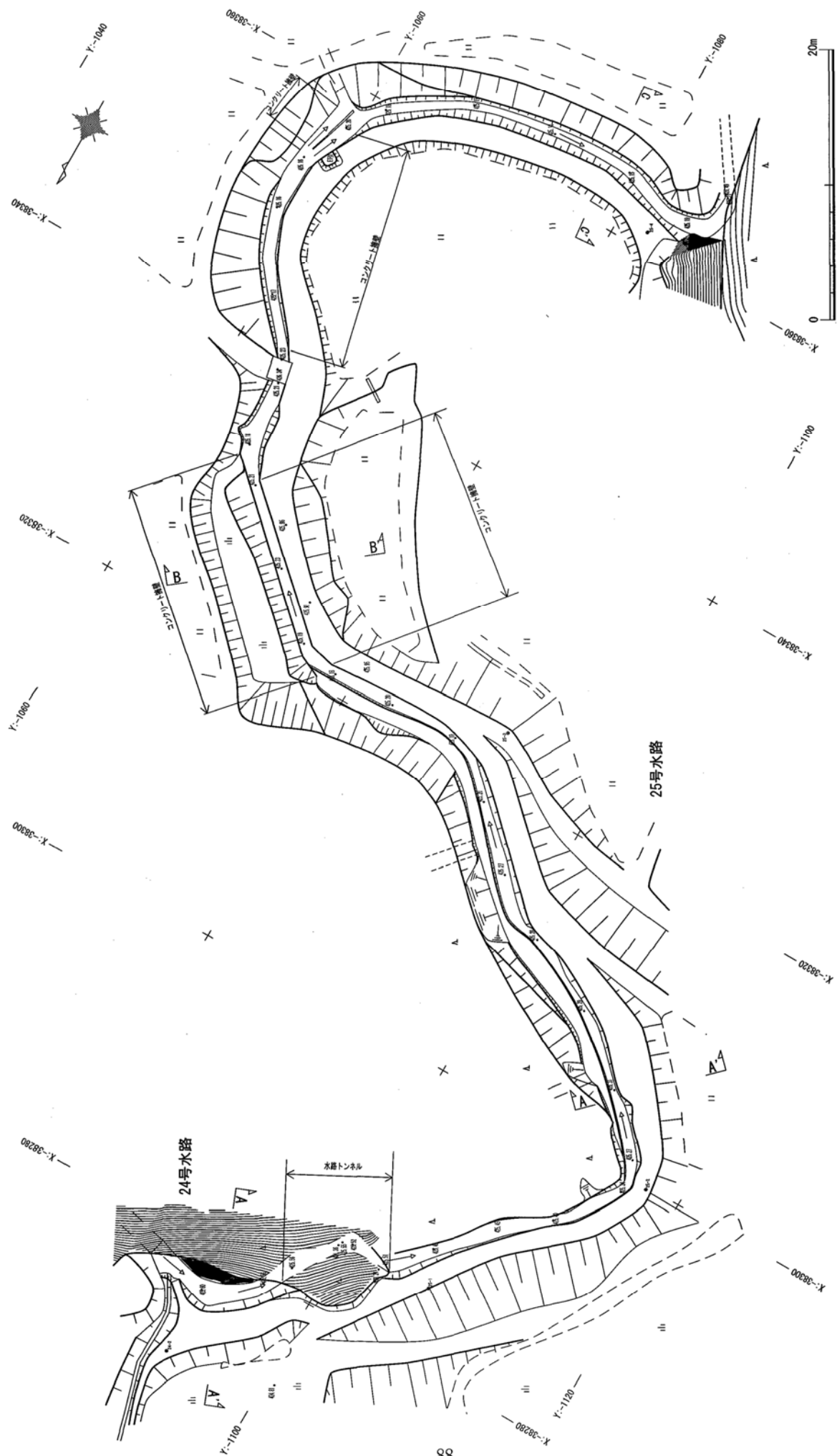
図 (PL) 50 通潤用水下井手24・25号水路 平面図 (S=1/400)
