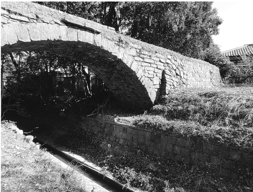
写真5-2-6 早鐘眼鏡橋 2 左岸下流側 袖石垣
