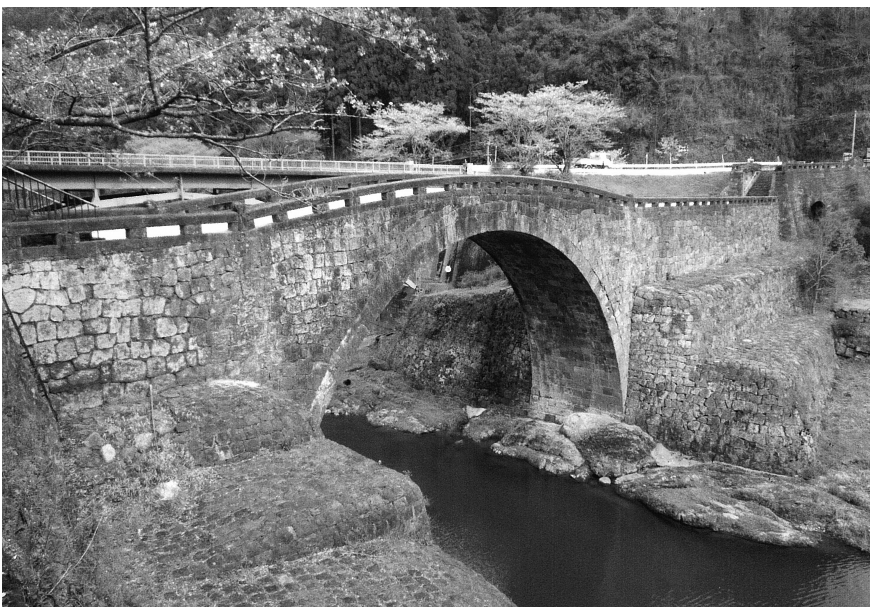
写真5-2-9 霊台橋 1
