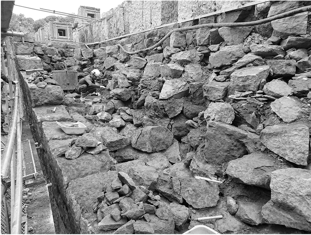
写真41 通潤橋 裏築と壁石（築石）①（令和元年（平成31年度）保存修理工事 / 裏築解体時）
