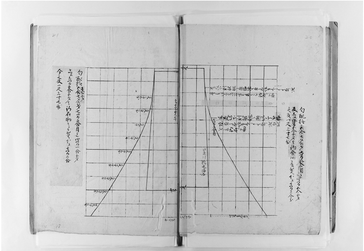
写真65 「通潤橋仕法書」② 「鞘石垣」の勾配に関する挿絵
