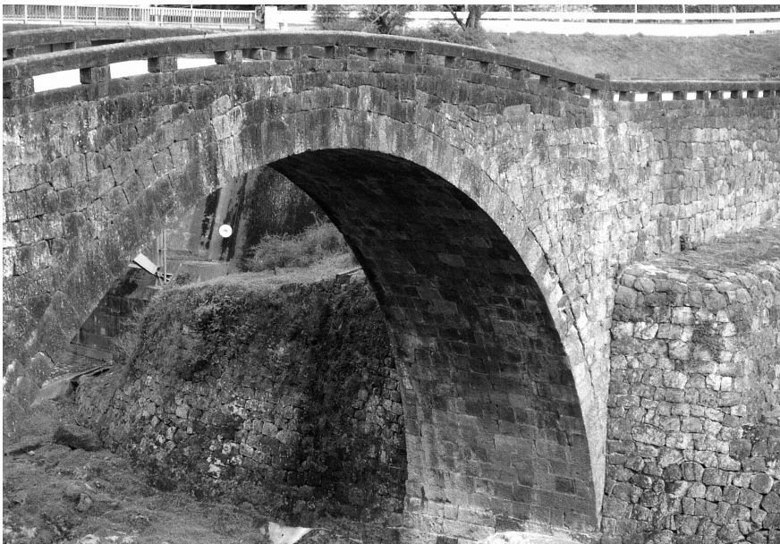
写真5-2-12 霊台橋 4
