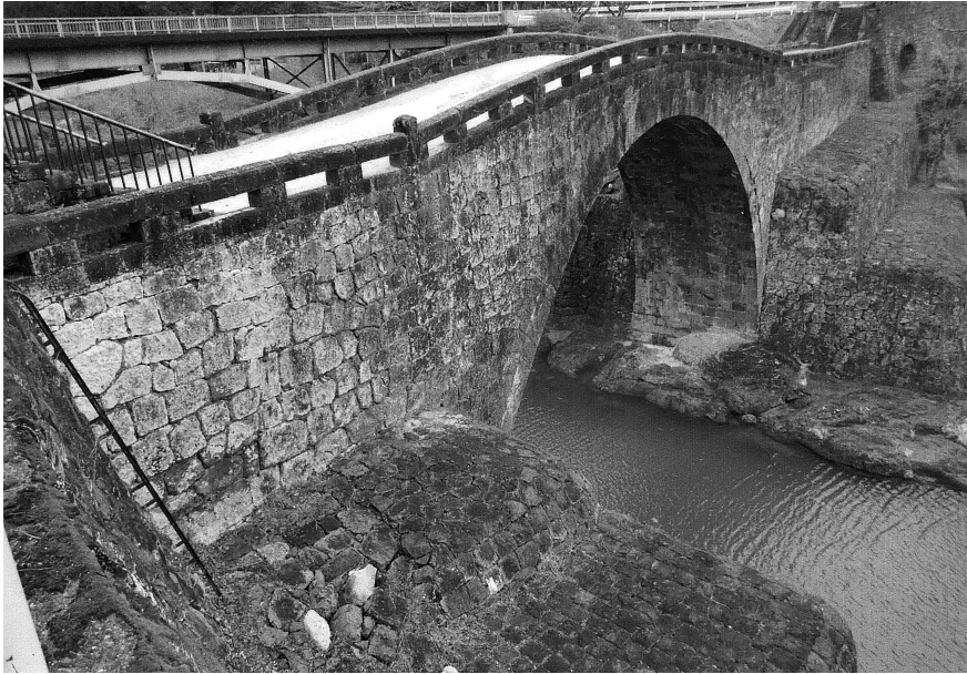
写真5-2-10 霊台橋 2
