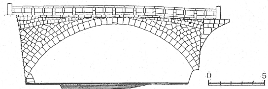
図5-2-18 湊川橋
