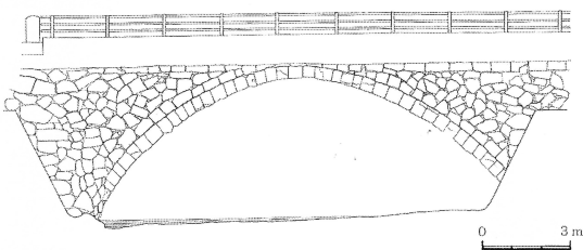
図5-2-16 三由目鑑橋 上流側立面図
