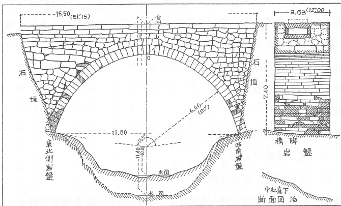
雄亀滝橋実測図
