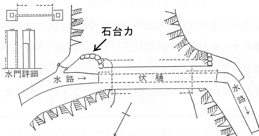
図5-2-15 雄亀滝橋 (著者加筆)
