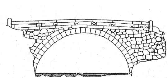
図5-2-17 赤松第一号目鑑橋 下流側立面図
