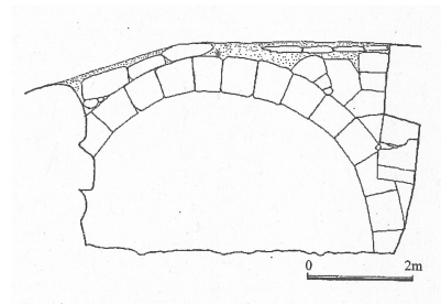
図5-2-19 鍛冶屋上橋
