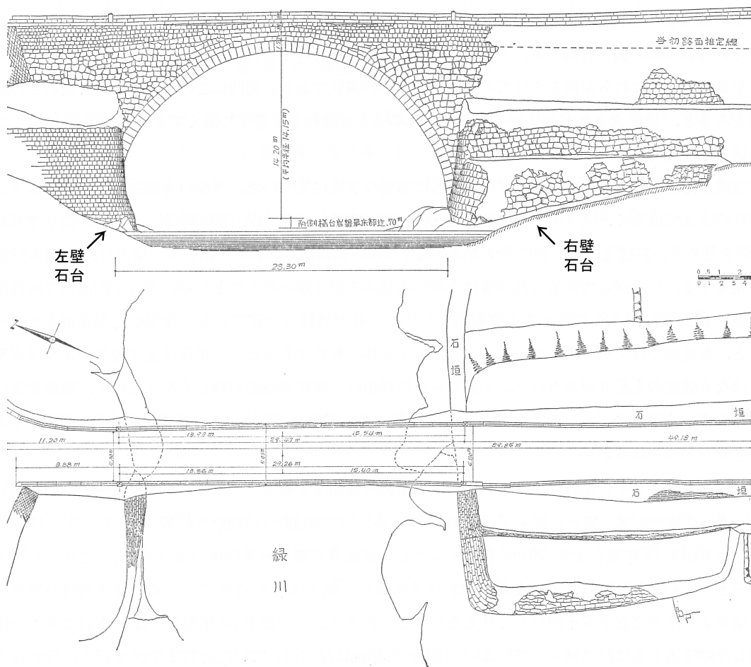
図5-2-21 霊台橋立面図・平面図 (著者加筆)
