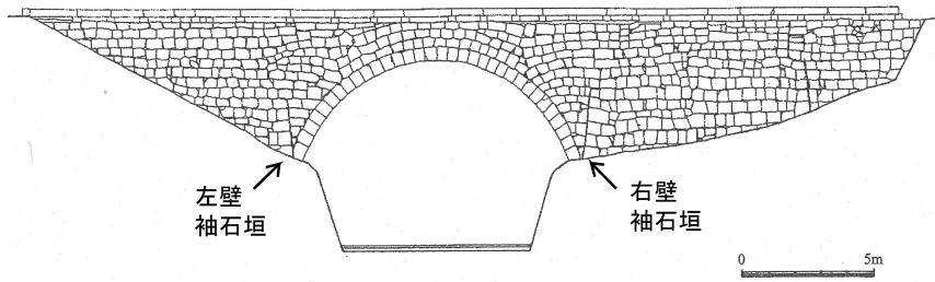
図5-2-20 小筵目鑑橋 (著者加筆)
