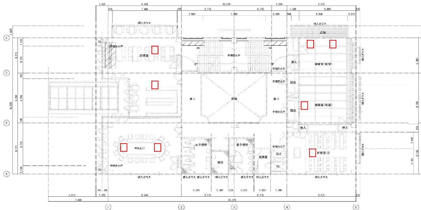
2階平面図
