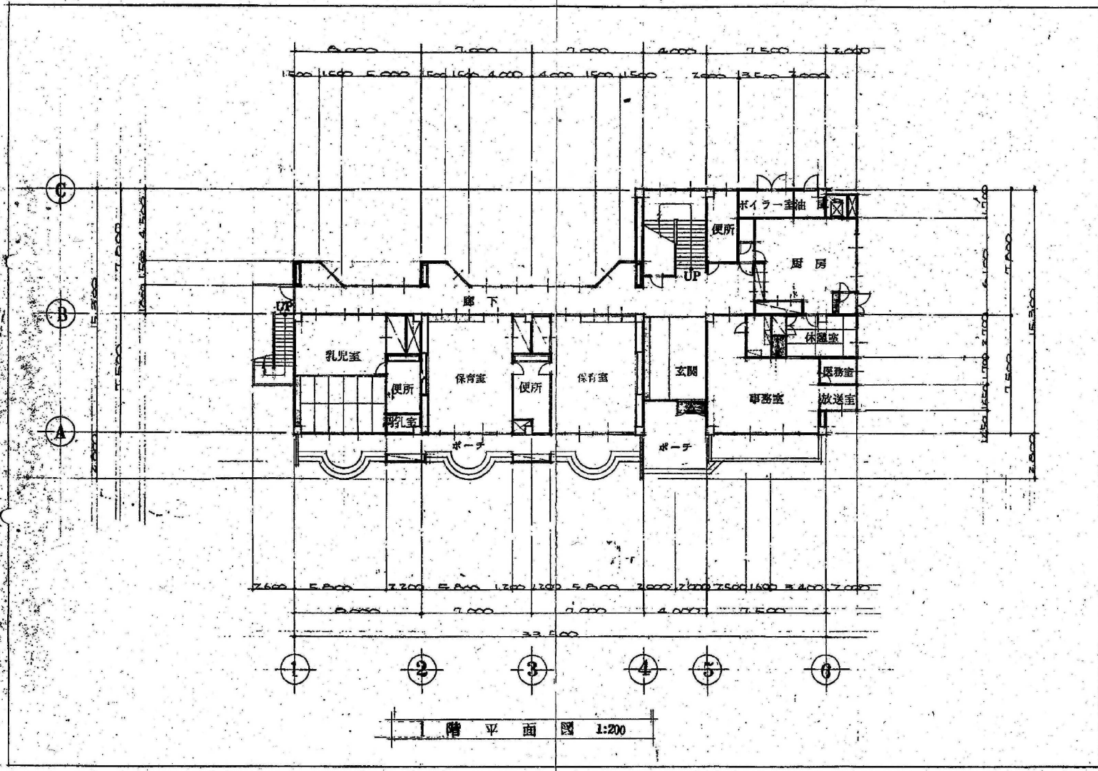
旧浜町保育園 1F平面図
