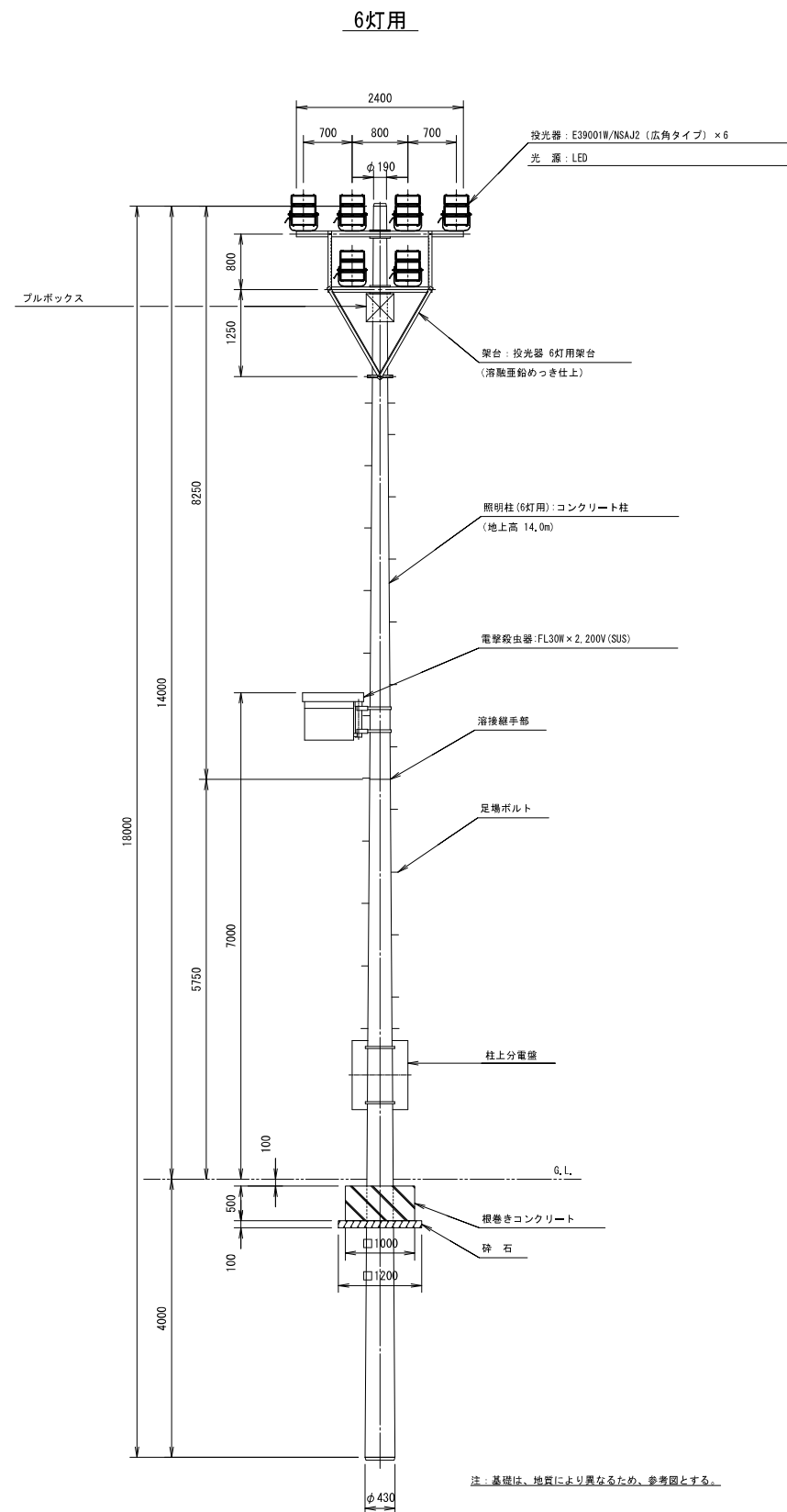
照明柱姿図 S=1/50
