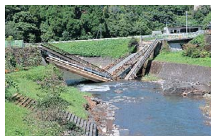
落橋した金内橋
