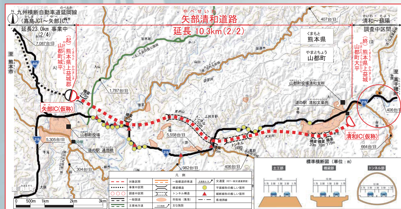
九州中央自動車道「矢部清和道路」計画図（九州地方小委員会資料より抜粋）
