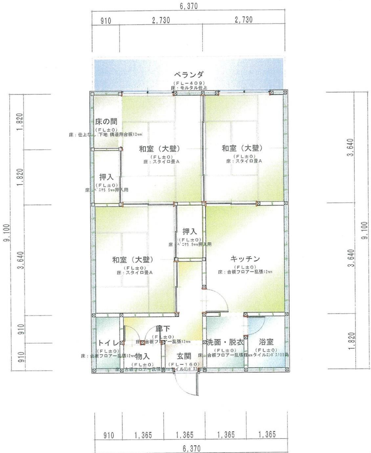
平面詳細図 1階
