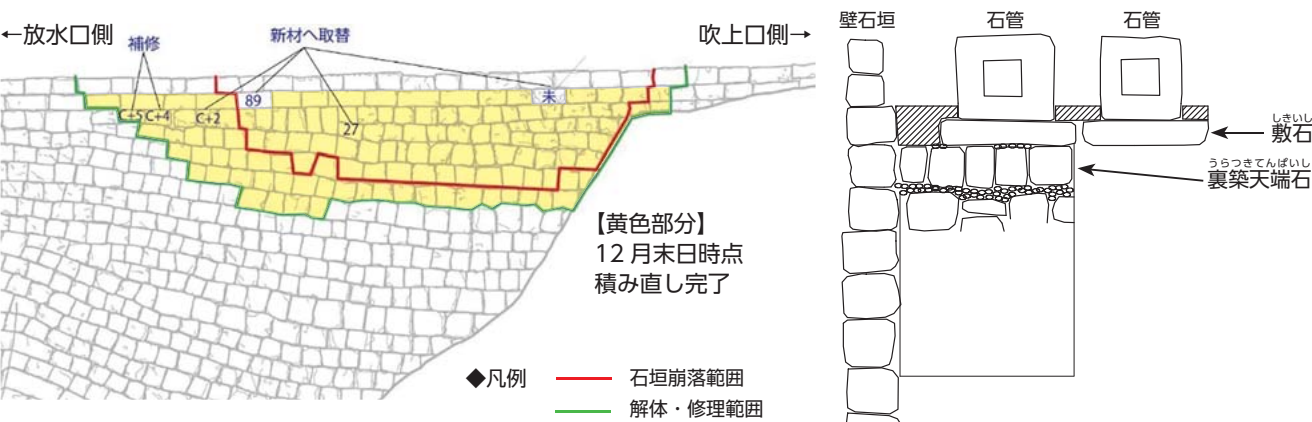
図1 石垣の修理範囲（立面図）
