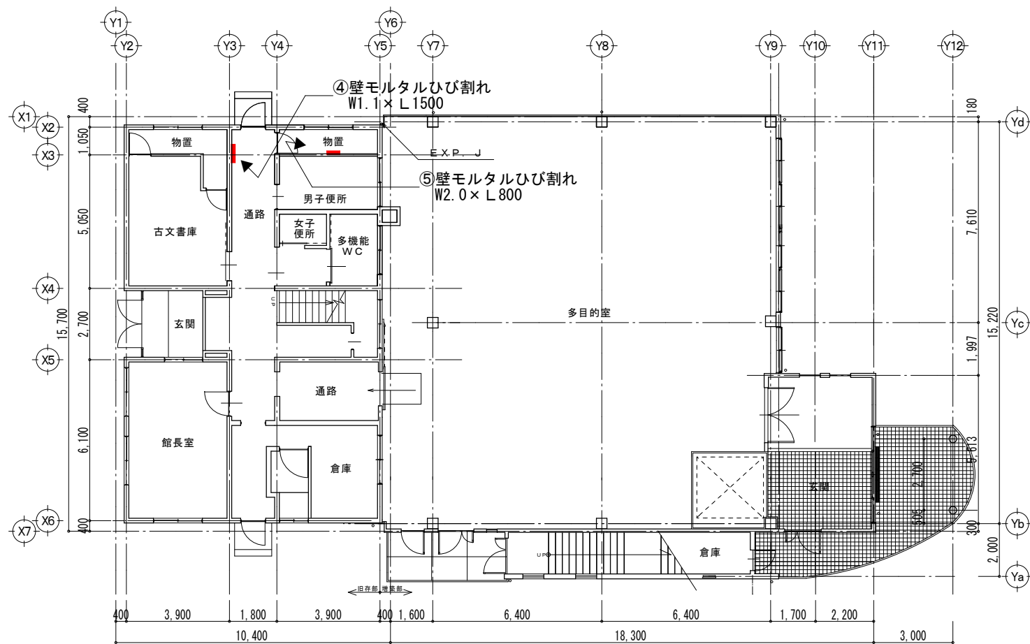
1 階平面図 S=1/200
