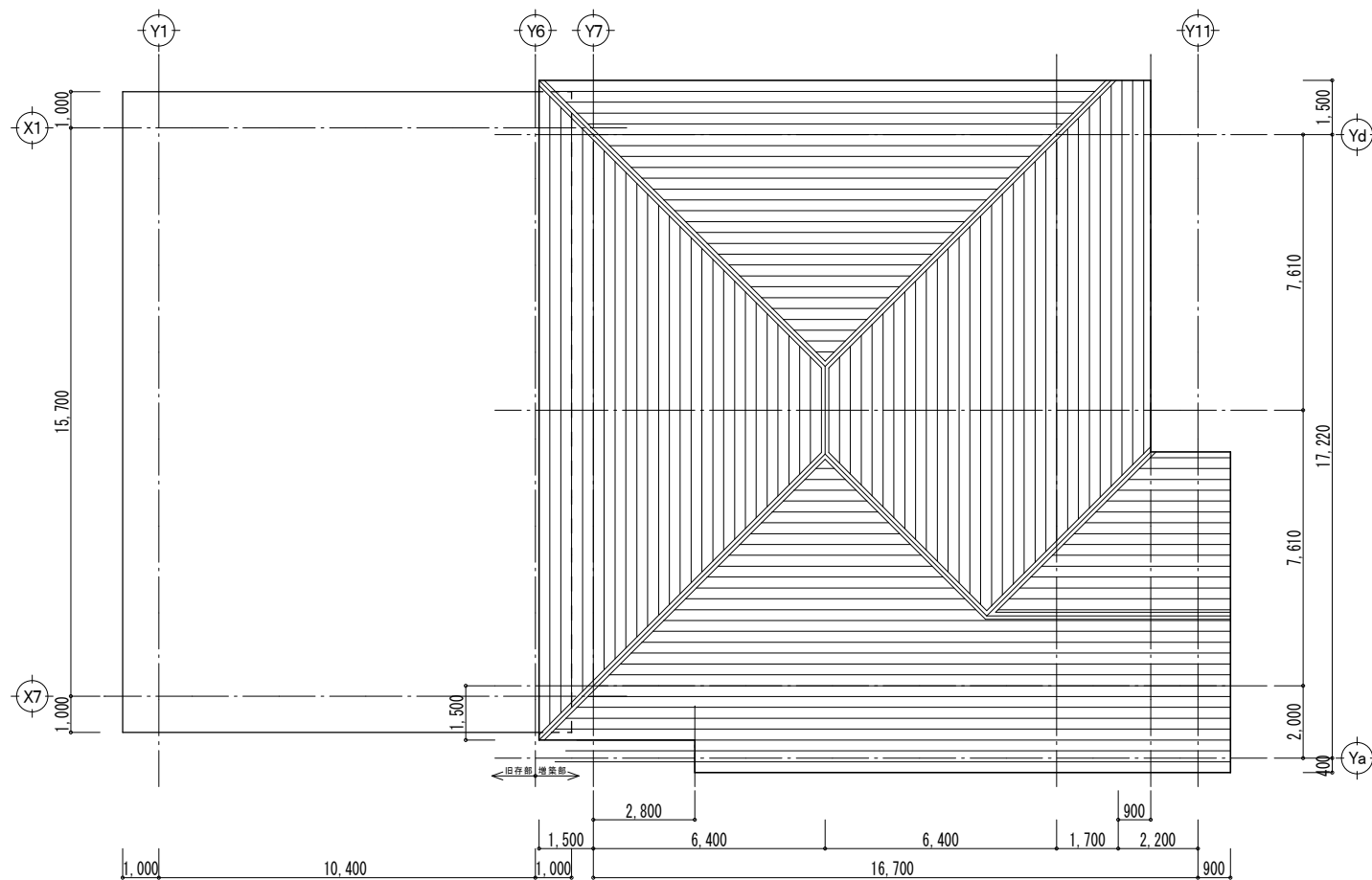
屋根伏図 S=1/200
